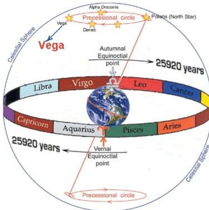
Слика 2. Прецесија Земљине осе
